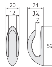
正面図・側面図(単位:mm)
