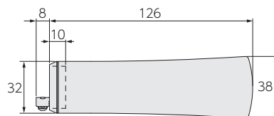
フィニアルB
