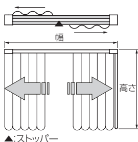
▲:ストッパー
