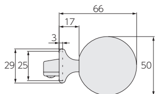
スタイリッシュフィニアルL
