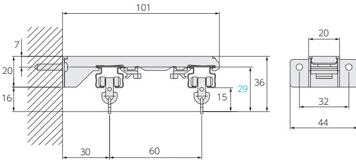
ワンタッチT型ダブルブラケット
