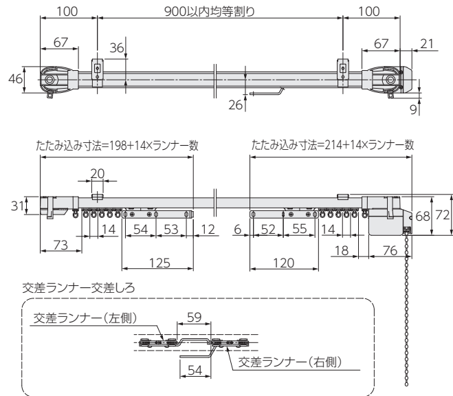
両開きの場合
