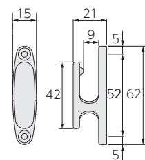
正面図・側面図(単位: mm)
