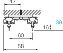
天井ダブルブラケット
