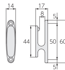
正面図・側面図(単位: mm)
