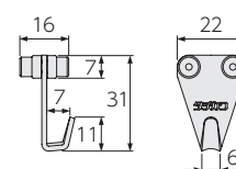
VPランナーフック25 (天井付け/先入れ)
