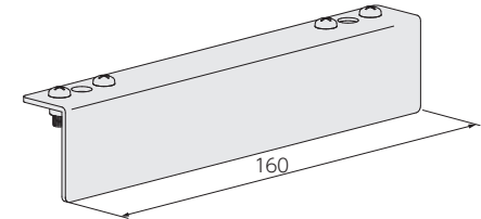
ストッパー (共通) (後付け)
