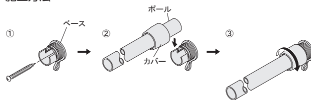
施工方法
