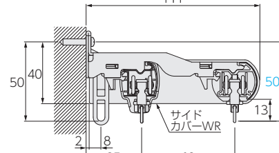
ワンタッチダブルブラケット+ サイドカバー-WR
