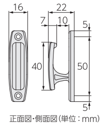
正面図・側面図(単位:mm)
