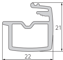
ホワイト(木目調)
