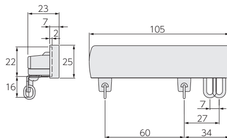
サイドカバー-W
