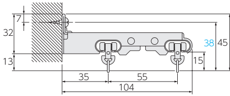
ワンタッチブラケットダブル正面付け (ブラケット幅:20)
