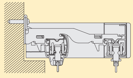
リターンホルダーをはずす
