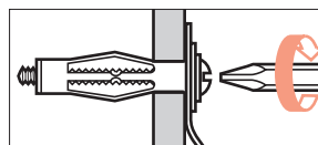
②共回り防止金具をセットして穴に差し込み、ネジの回転が重たくなるまで十分に締め付けます。
