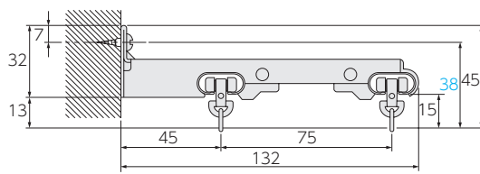
ワンタッチブラケットロングダブル正面付け (住宅公団指定仕様: AI-911C型) (ブラケット幅:20.8) (旧jl-801C型)
