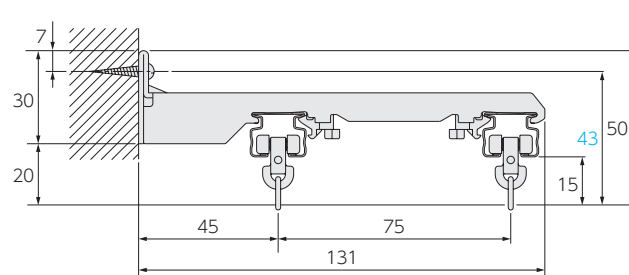
ワンタッチロングダブルブラケット (ブラケット幅:21)
