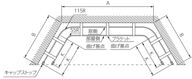
ダブル付けV5取付け例
