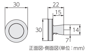
正面図・側面図(単位:mm)
