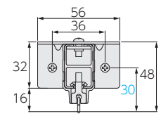
フリーソケット
