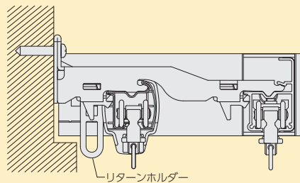
リターンホルダーをずらして付ける
