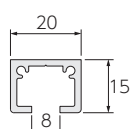
VP-30レール
