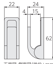
正面図・側面図(単位:mm)
