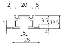
VP-30Aレール (9.5mm)
