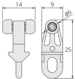
後入れランナー
