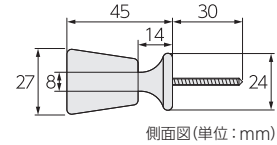
側面図(単位:mm)
