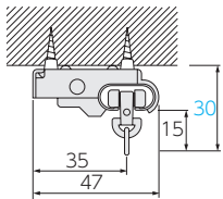
ワンタッチブラケット シングル天井付け (ブラケット幅:20)
