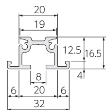
VP-30Bレール (12.5mm)
