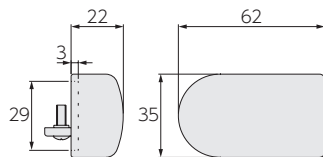
ウッドサイドカバー SR
