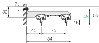
ロングダブルブラケット
