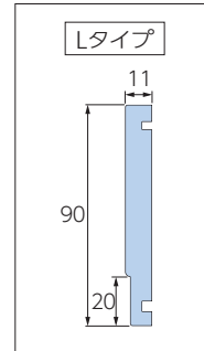
断面図 [単位:mm]
