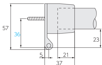
ソケット
