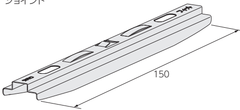
ジョイント
