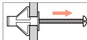
③共回り防止金具をはずしネジをゆるめて抜き取ります。
