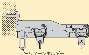
①リターンホルダーを付ける
