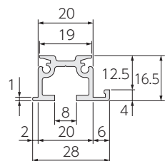
VP-30Aレール (12.5mm)
