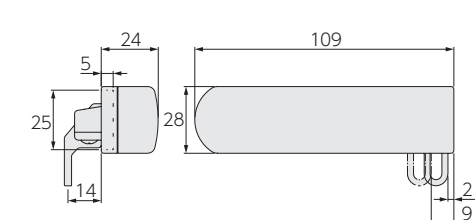
サイドカバー WR
