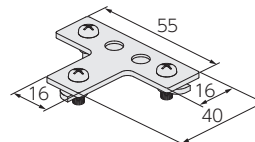
T型金具
