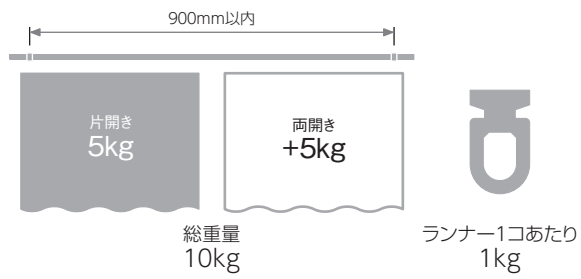
Eランナー
