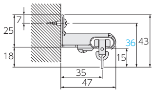
ワンタッチブラケットダブル正面付け (ブラケット幅:20)
