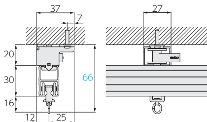
天井付け用ブラケット
