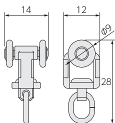
ランナー
