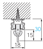
天井直付け
