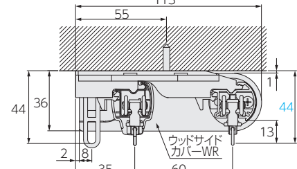
天井ダブルブラケット+ ウッドサイドカバー-WR
