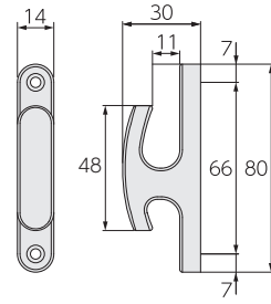
正面図・側面図(単位:mm)
