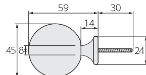
側面図(単位:mm)
