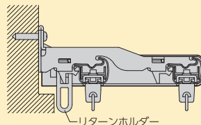
②リターンホルダーをずらして付ける
