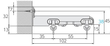
ダブル正面付け (ブラケット幅:20)
