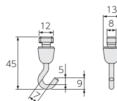
VPランナーフック25 (天井付け/先入れ)
