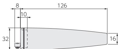
フィニアルA
