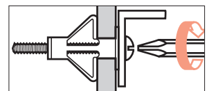
④取付け物をセットし、ネジを締め付け施工完了。
