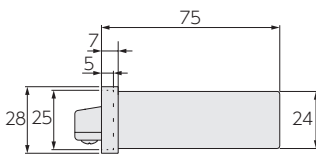
サイドカバー WR
