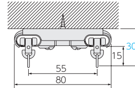
ダブル天井付け (ブラケット幅:20)
