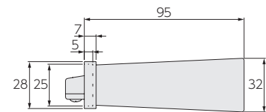
サイドカバー SR
