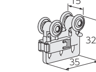
共通マグネットランナー (片開)
